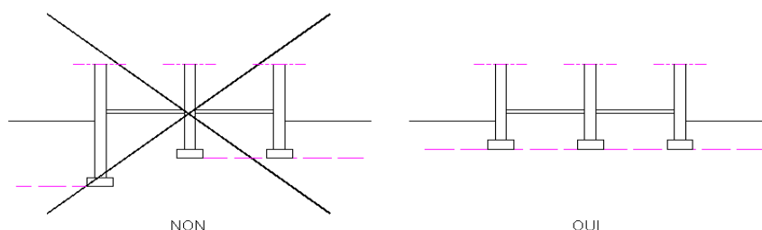
Plan d'assise des fondations
